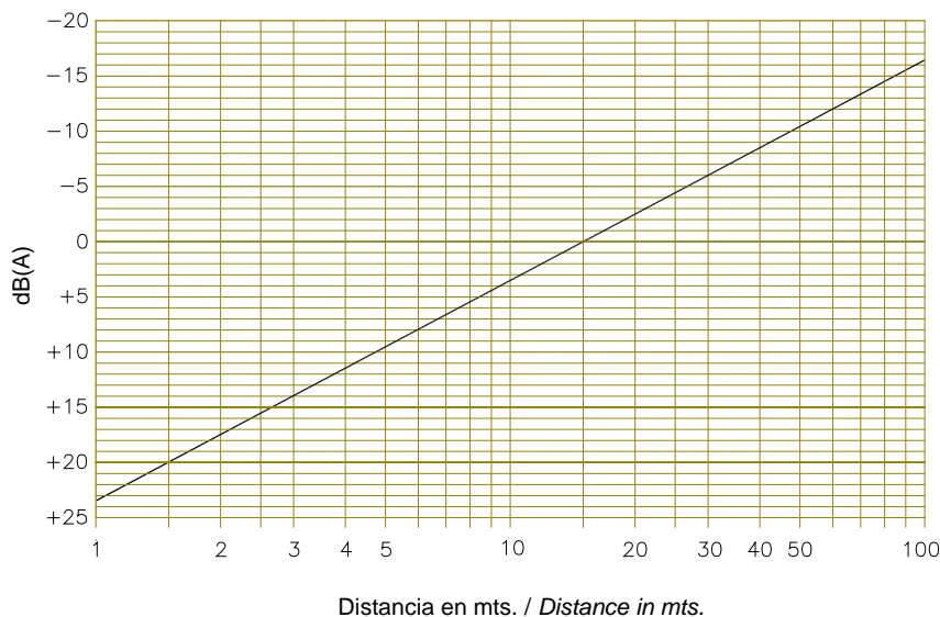
Variación nivel sonoro con la distancia / Noise level variation with the distance
